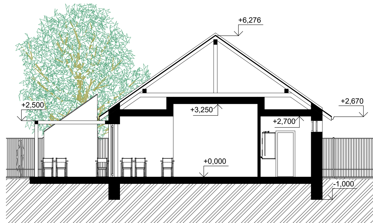
ŘEZ B-B
