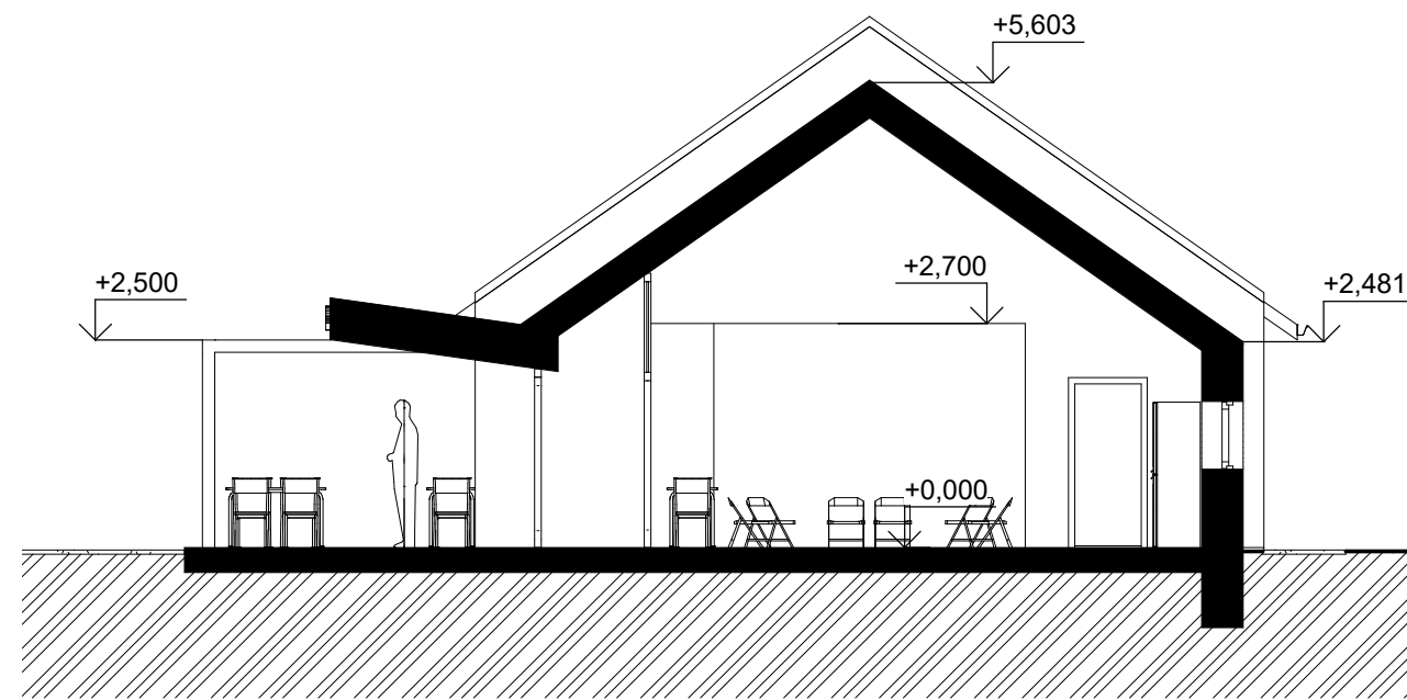
ŘEZ B-B
